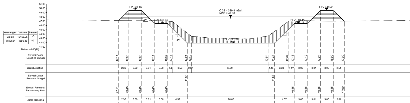
CROSS SECTION 1+200 SKALA : 1:40
