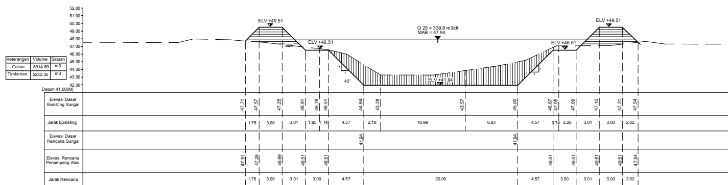
CROSS SECTION 1+400 SKALA : 1:40
